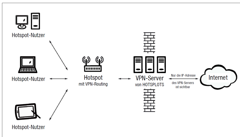
Abbildung 2: Funktionsdiagramm eines Hotspots mit VPN-Routing
